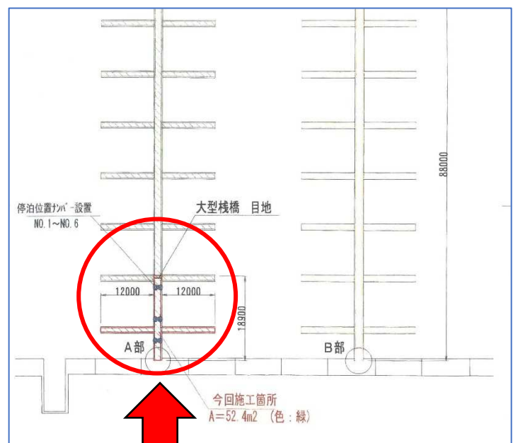
大型棧橋 A の通路部分の一部
