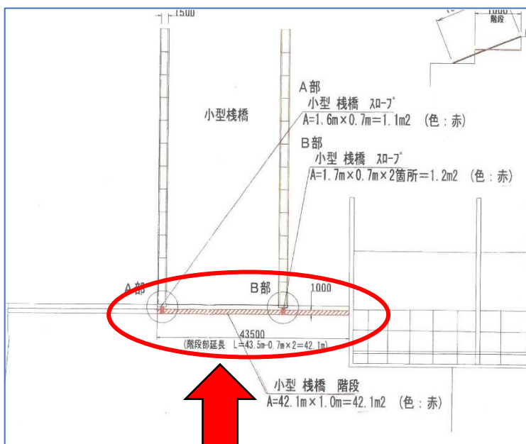
小型棧橋階段部分
